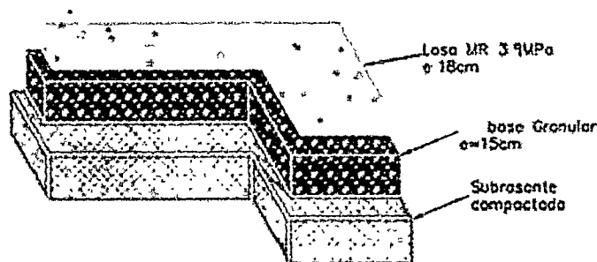
Ilustración 5. Estructura de pavimento BUENAVISTA (40QN06)
