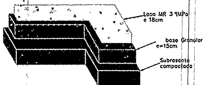
Ilustración 5. Estructura de pavimento BUENAVISTA (40QN06)
