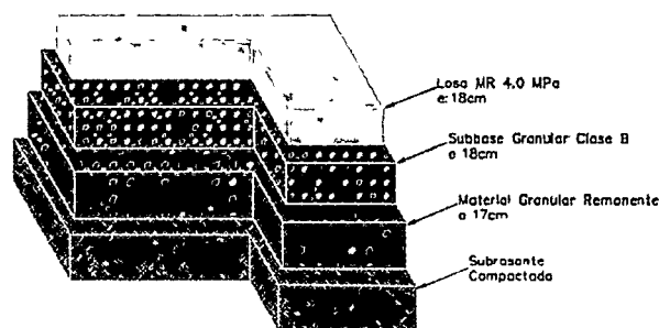
Ilustración 6. Estructura de pavimento BARAYA – PUERTO SAMARIA (210BQN02-1)
