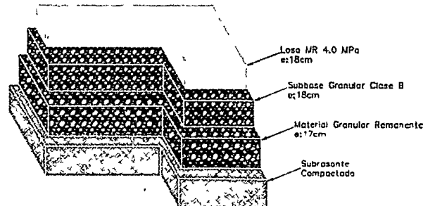
Ilustración 6. Estructura de pavimento BARAYA – PUERTO SAMARIA (210BQN02-1)
