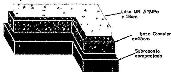
Ilustración 5. Estructura de pavimento BUENAVISTA (40QN06)
